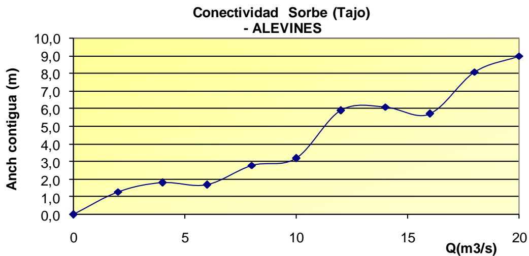
Figura 9. Gráfica de anchura de paso caudal por tramo unidimensional
